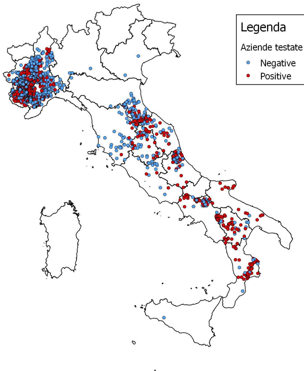
Figura 18: distribuzione spaziale per esito IBR delle 3.235 aziende testate
